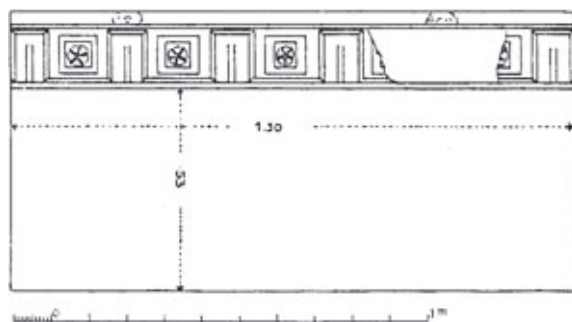
Abb. 160: Gesimsplatte, Unteransicht (nach Wilberg)
