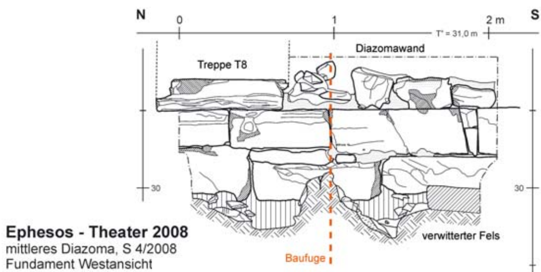
Abb. 232: Mittleres Diazoma, S 4/2008, Fundament, W-Ansicht
