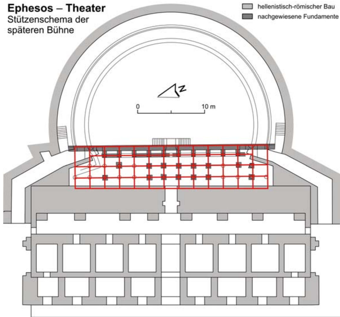
Abb. 154: Späte Bühne: Rekonstruktion des Stützenschemas
