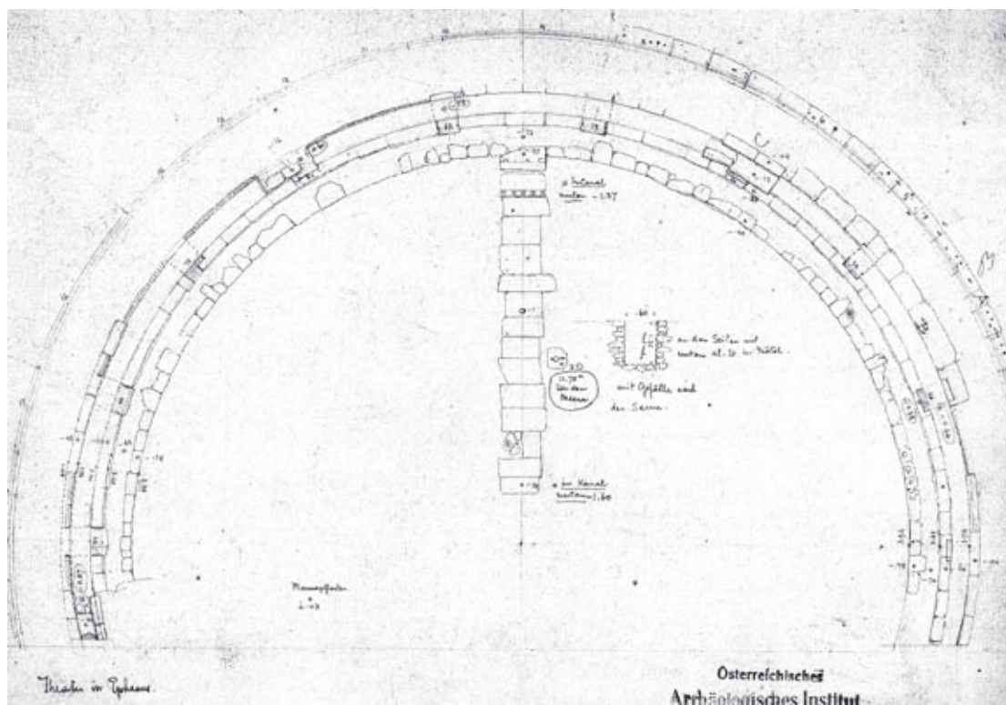
Abb. 162: Orchestra, Handzeichnung (Aufnahme um 1900)
