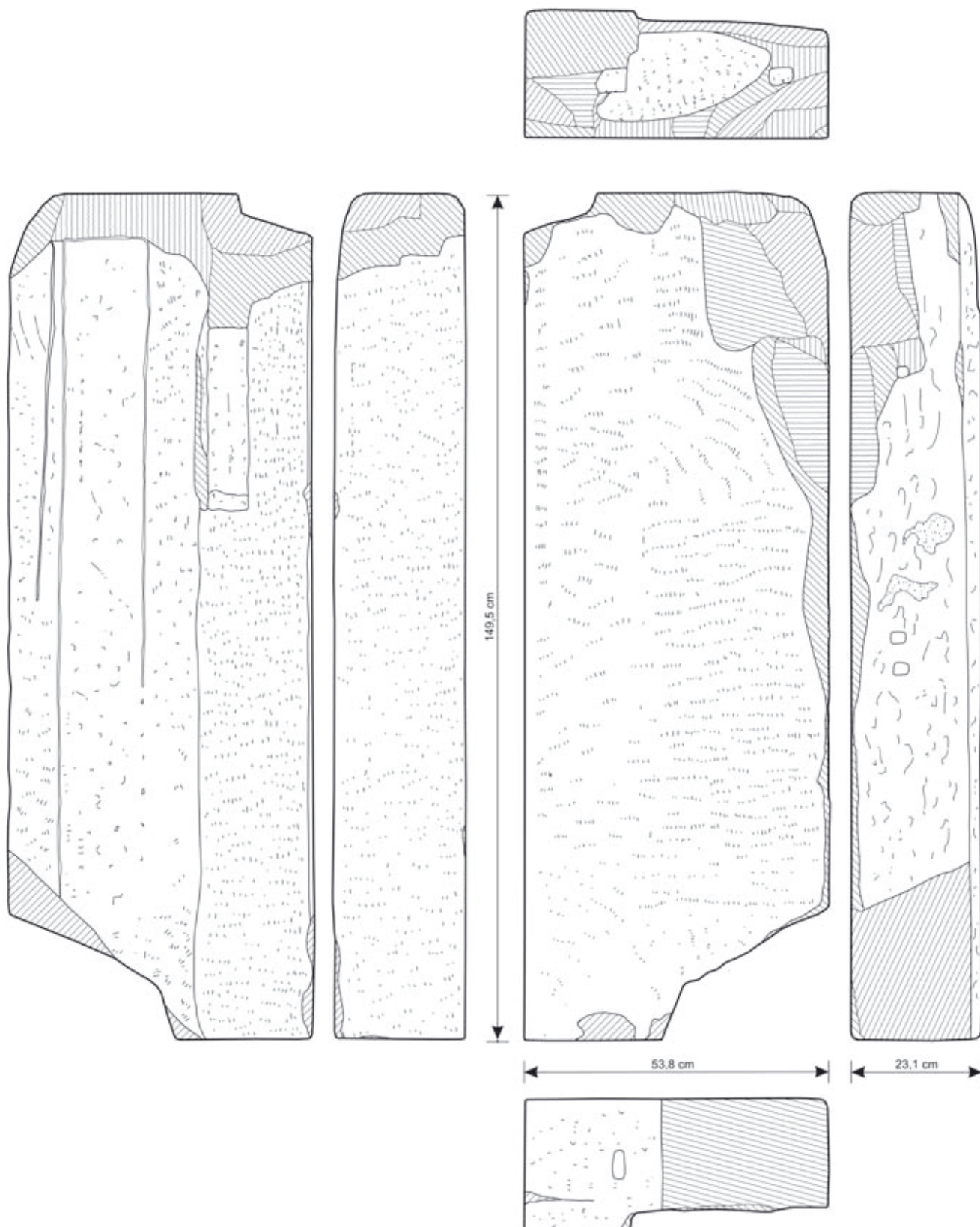
Abb. 158: Pfeiler des kaiserzeitlichen Proskenion
