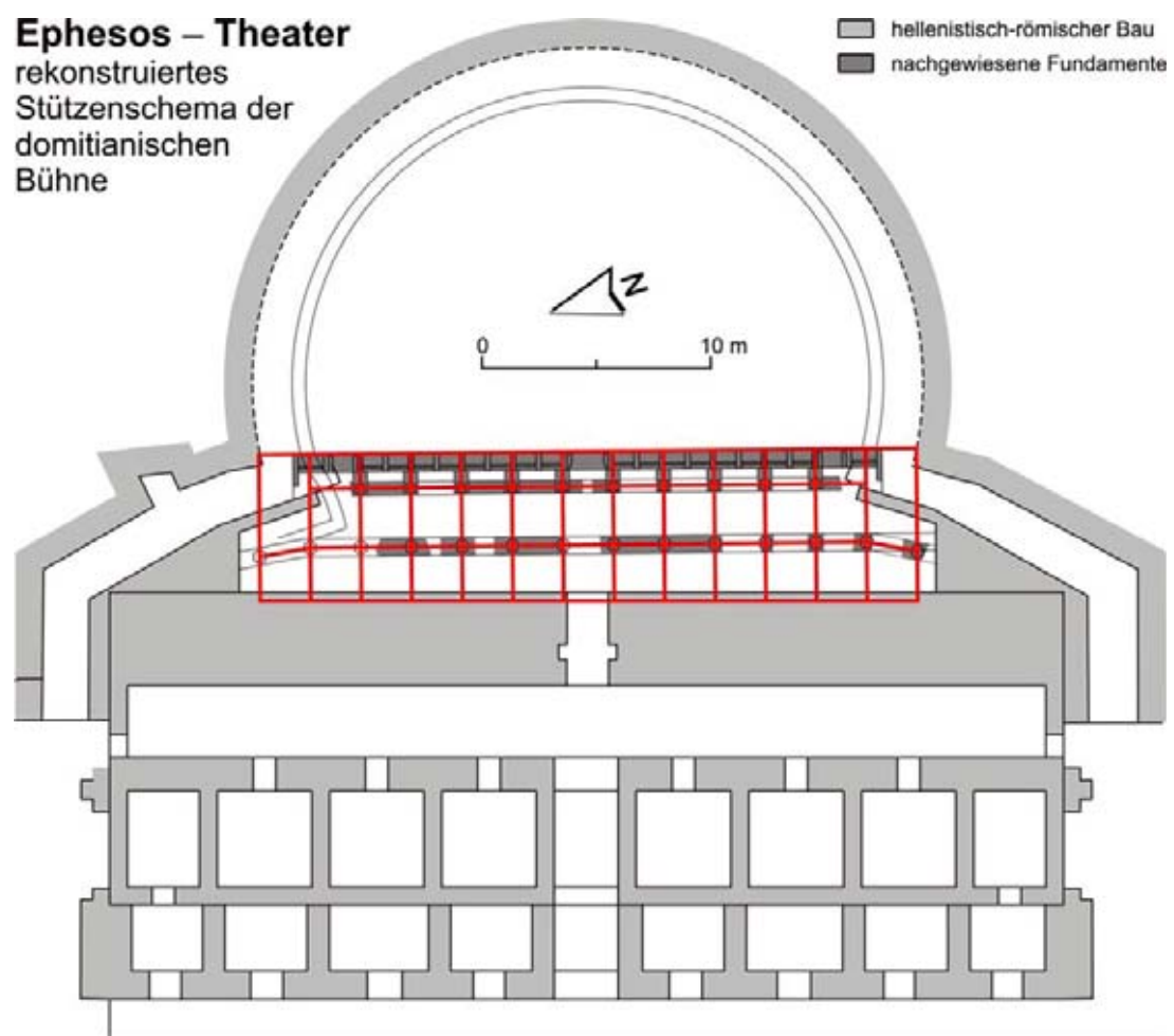
Abb. 153: Flavische Bühne: Rekonstruktion des Stützenschemas
