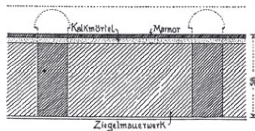
Abb. 157: Rekonstruktion des Pfeilerjochs nach dem Umbau (nach Wilberg)
