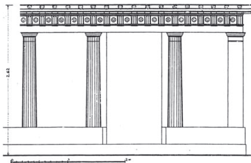
Abb. 161: Aufbau des Proskenion
