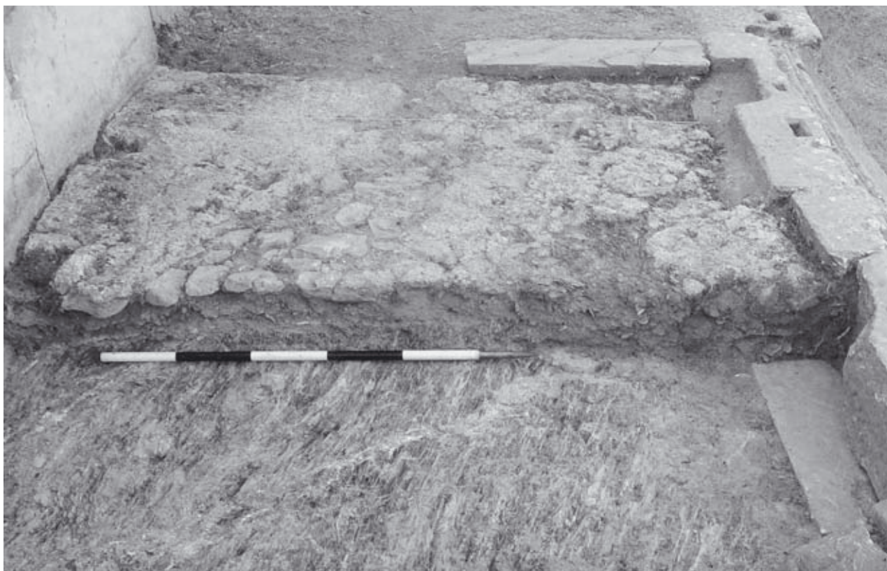
Abb. 171: Orchestra, S 3/2004, Detail Mörtelbett für opus-sectile -Boden, von N
