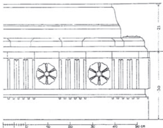
Abb. 159: Gebälk des Proskenion (nach Wilberg)
