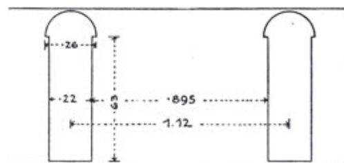
Abb. 156: Rekonstruktion des Pfeilerjochs (nach Wilberg)
